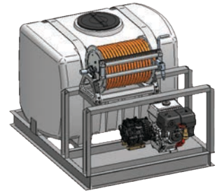
200 GALLON SKID
