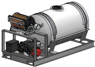
300 GALLON SKID
