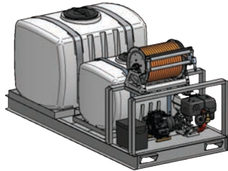
200/100 GALLON SKID
