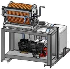
50 GALLON SKID
